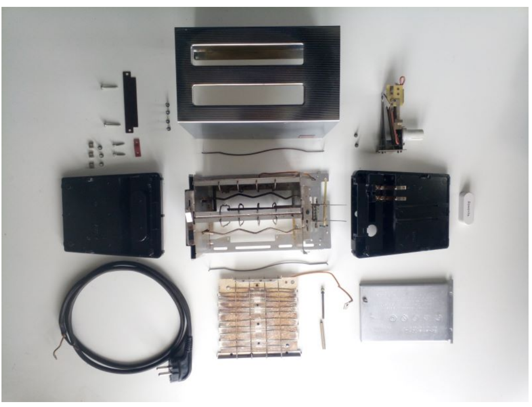
Zerlegbar bis zur letzten Schraube.
