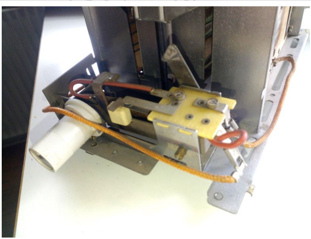
Analoge Zeitsteuerung.
