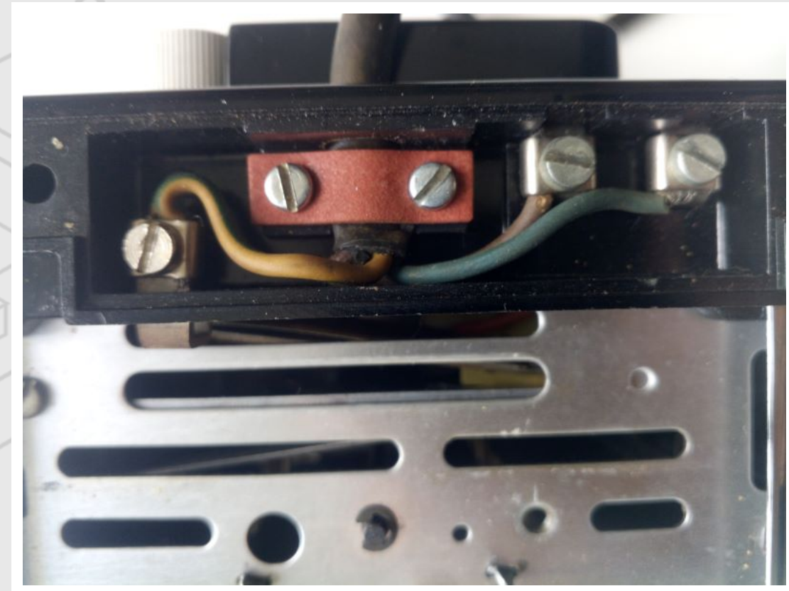
Übersichtliche Anschlüsse. Kabeltausch möglich.
