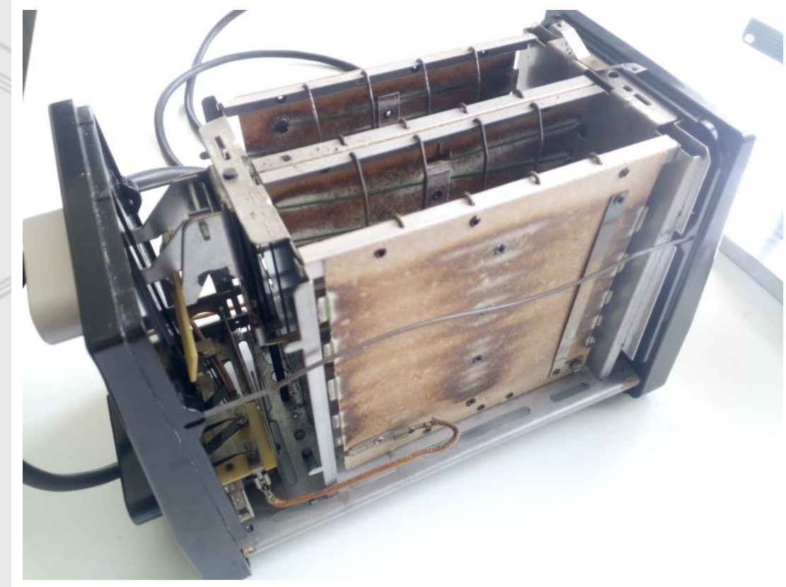
Heizplatten können ausgeschraubt und getauscht werden.
